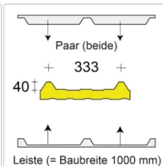
Leiste (= Baubreite 1000 mm)
